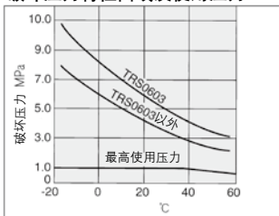
破坏压力特性曲线及使用压力
