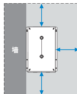
IDF100F的设置空间 (在左面贴墙壁安装例)
