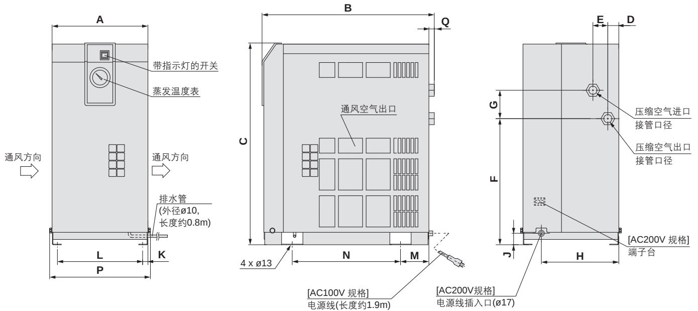
尺寸表
