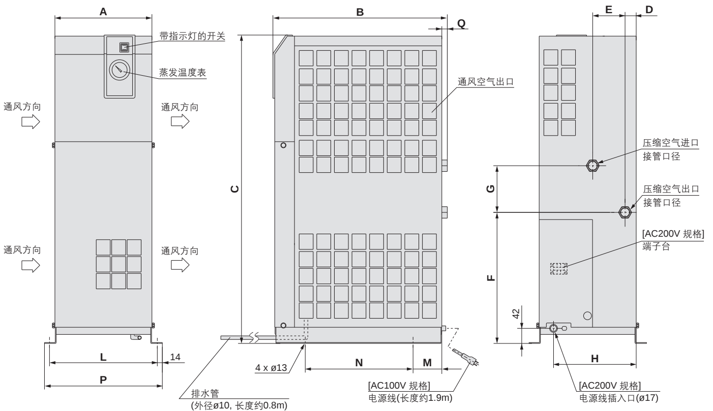
尺寸表
