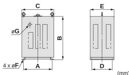
规格/尺寸表
