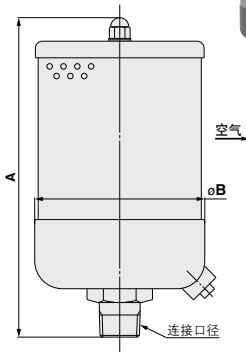
AMV3・6・15・37
