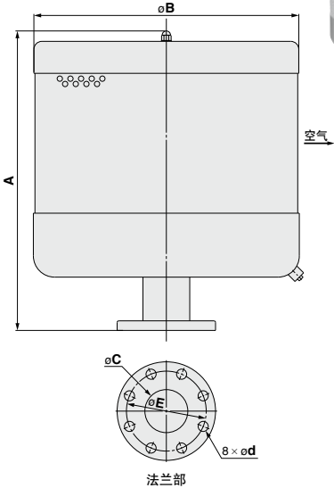
AMV75・160
