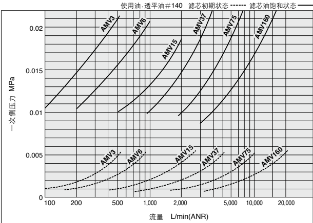
AMV3・6・15・37
