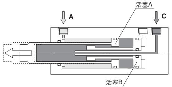
第一段伸出
