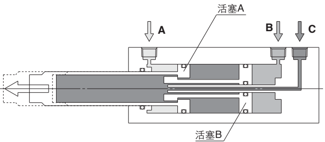
第二段伸出
