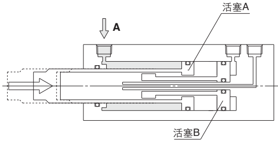
第一段缩回
