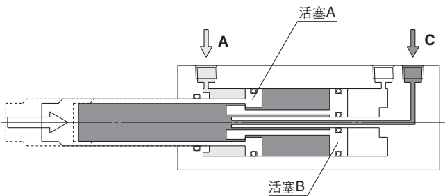
第二段缩回
