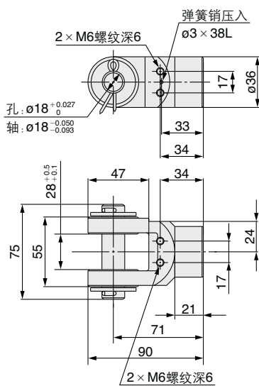
双肘接头
