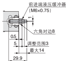
前进端
