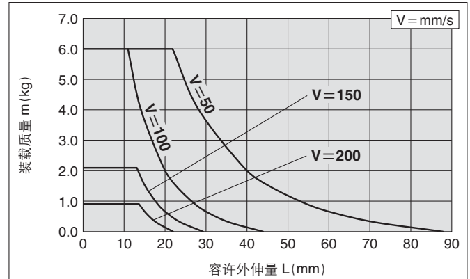
MXQ20(A)-100、150Z□
