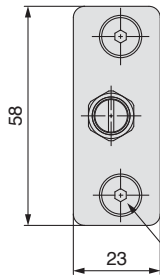
MXQA-JT12~JT25 の場合 MXQA-JT8 の場合
