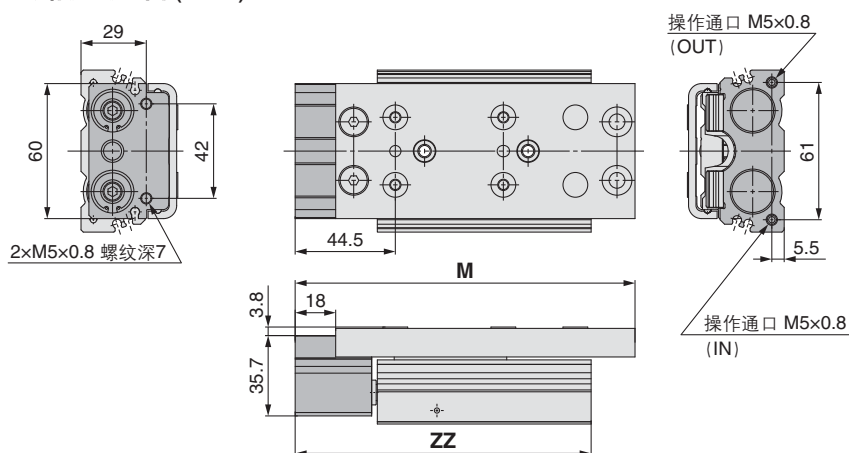
尺寸表
