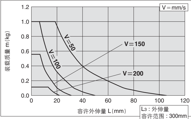
MXQ6B-50、75Z□
