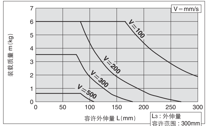
MXQ25(A)-50、75Z□
