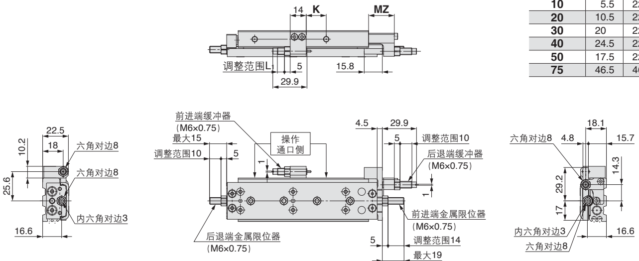
尺寸表
