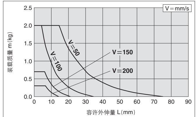
MXQ12(Δ)-40、50Z□
