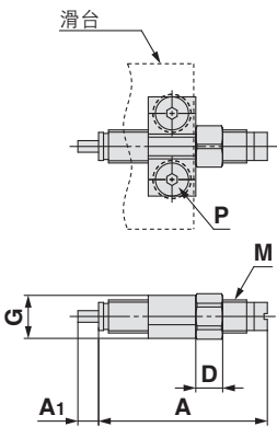
MXQA-JS8 の場合
