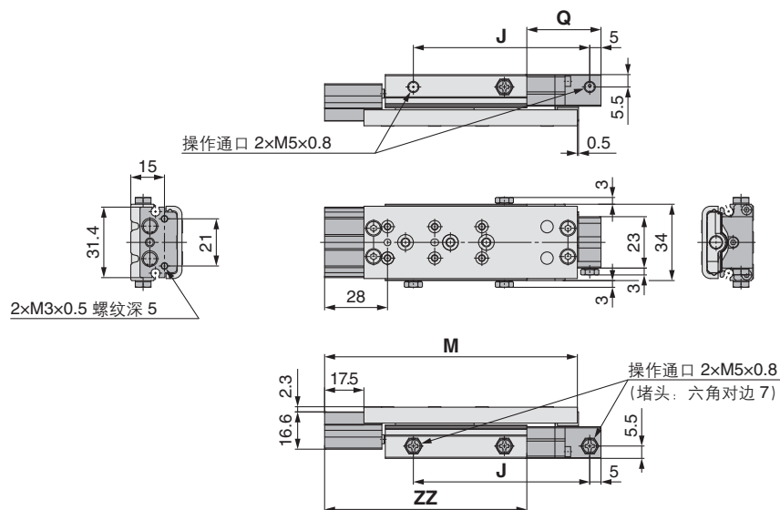
尺寸表
