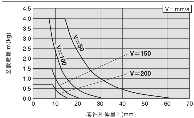
MXQ16(A)-75Z□
