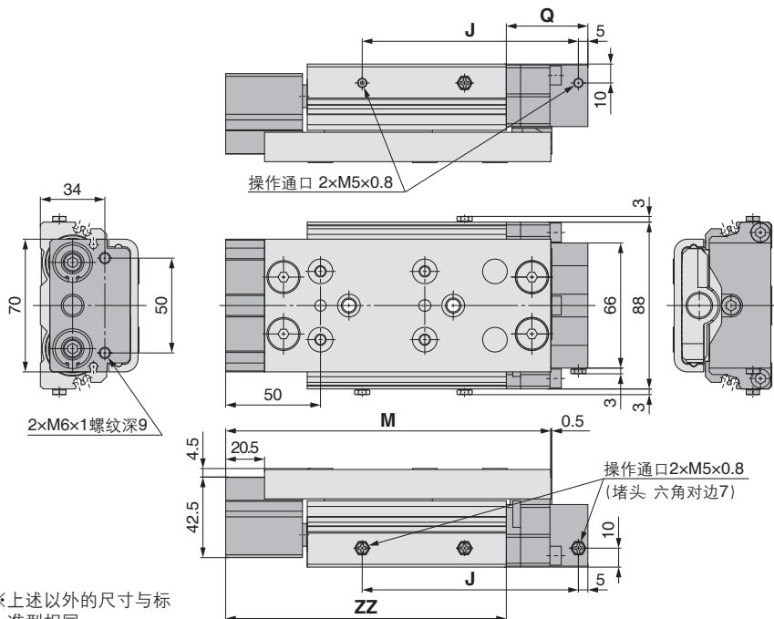
尺寸表
