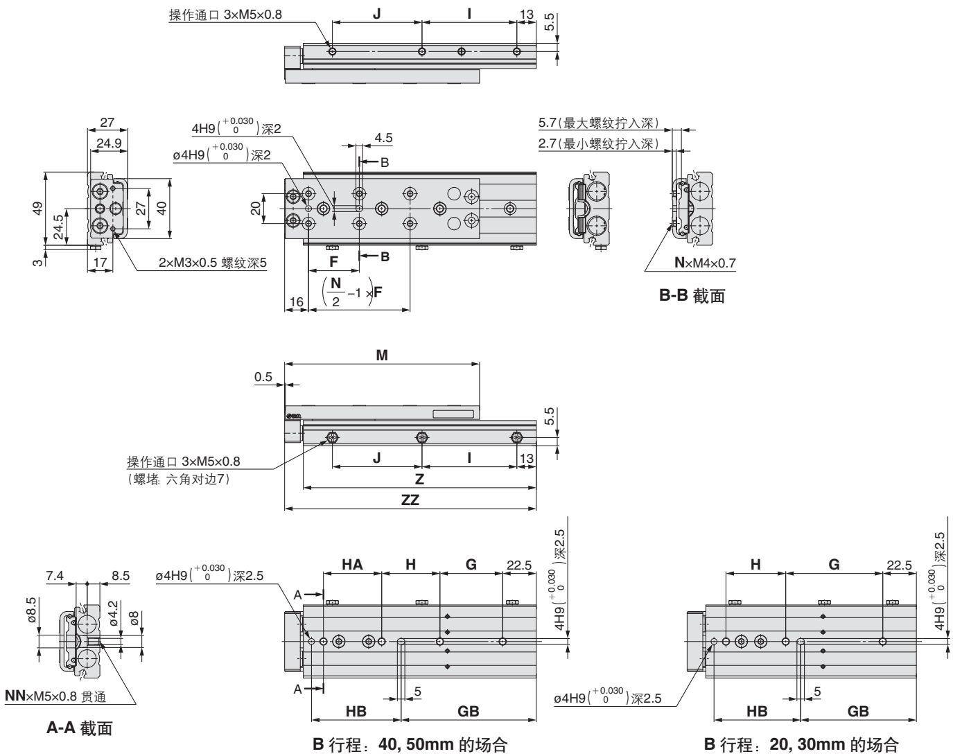
尺寸、质量表
