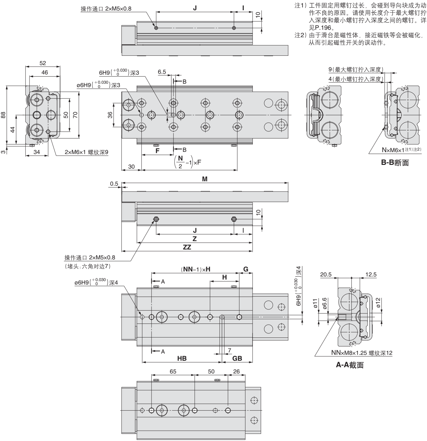
尺寸表 MXQ25A-75Z的底面图
