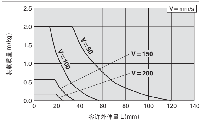
MXQ16(A)-10、20、30Z□
