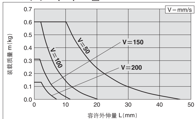
MXQ8 A C -40Z□
