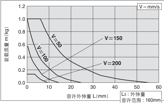
MXQ6B-40Z□
