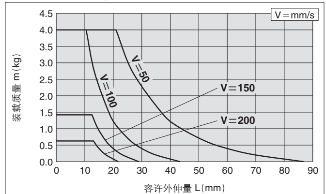
MXQ16(A)-100、125Z□
