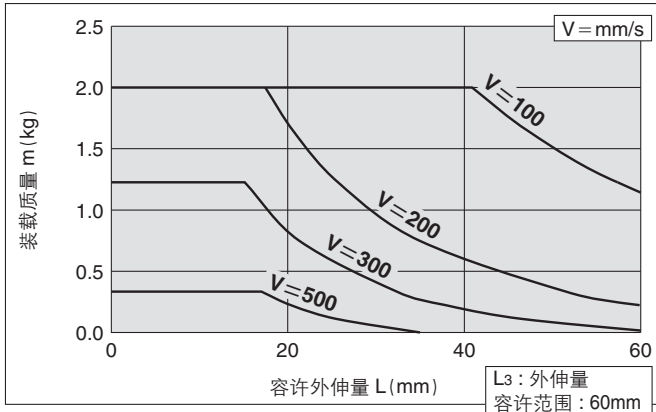
MXQ12(Δ)-75、100Z□
