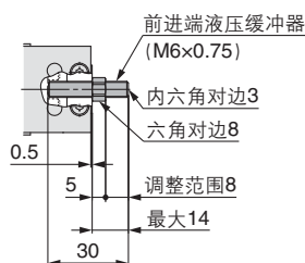
前进端
