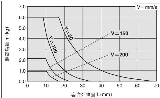
MXQ20(A)-75Z□
