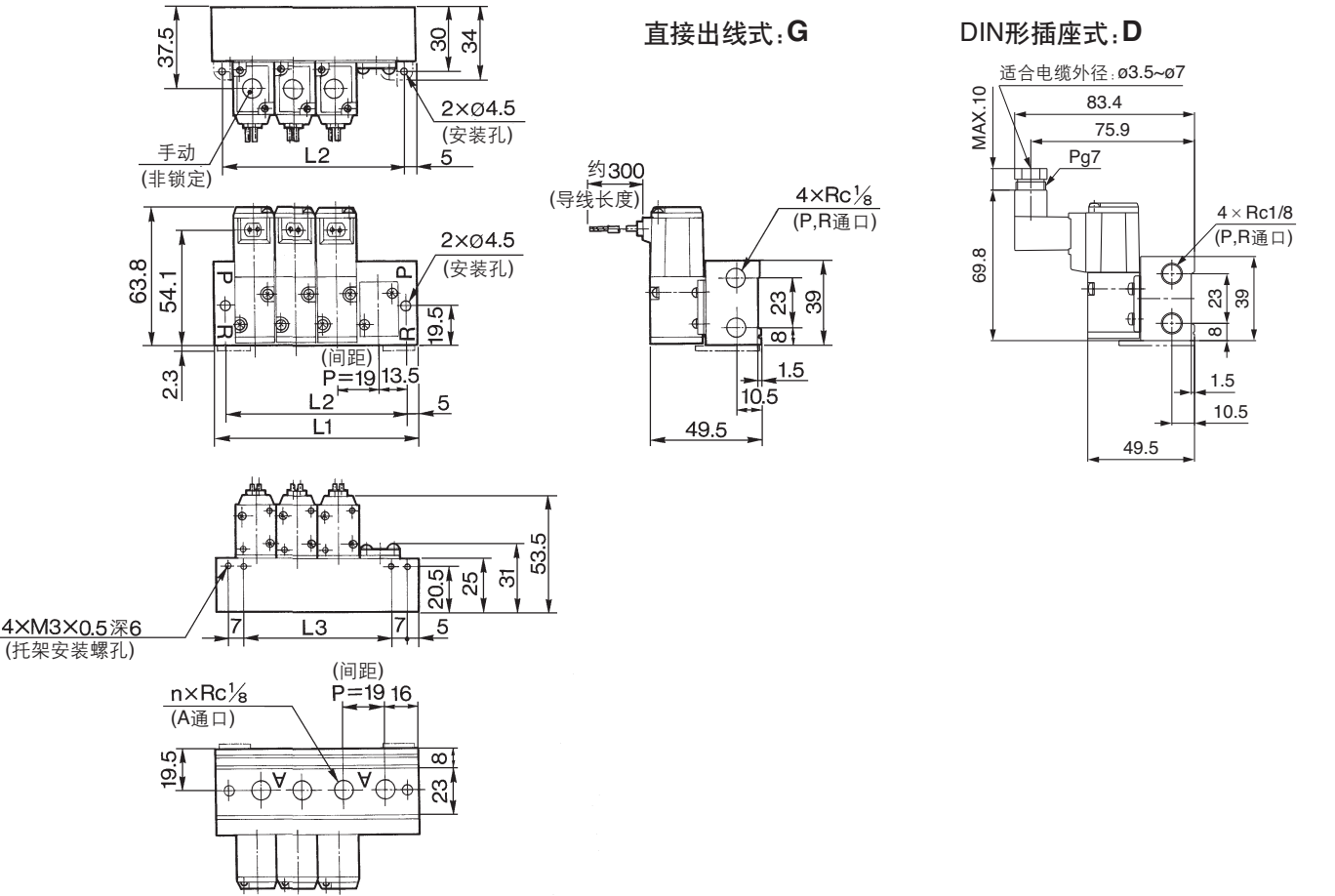
L: 尺寸表
