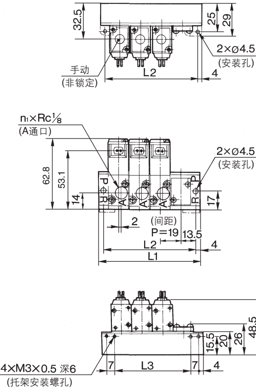
L: 尺寸表
