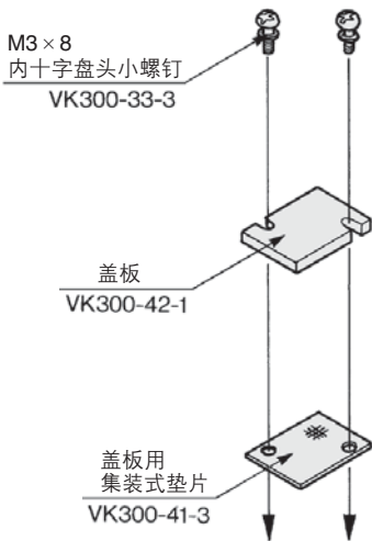
盖板组件: VK300-42-1A
