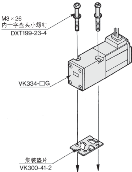
3通底板配管型: VK334
