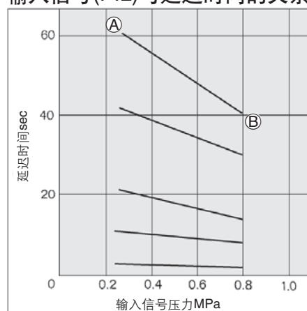
输入信号(PIL)与延迟时间的关系
