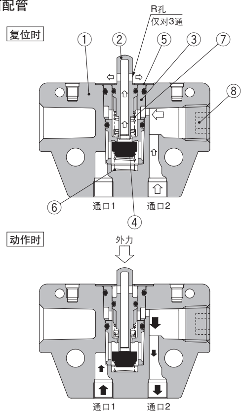
底面配管
