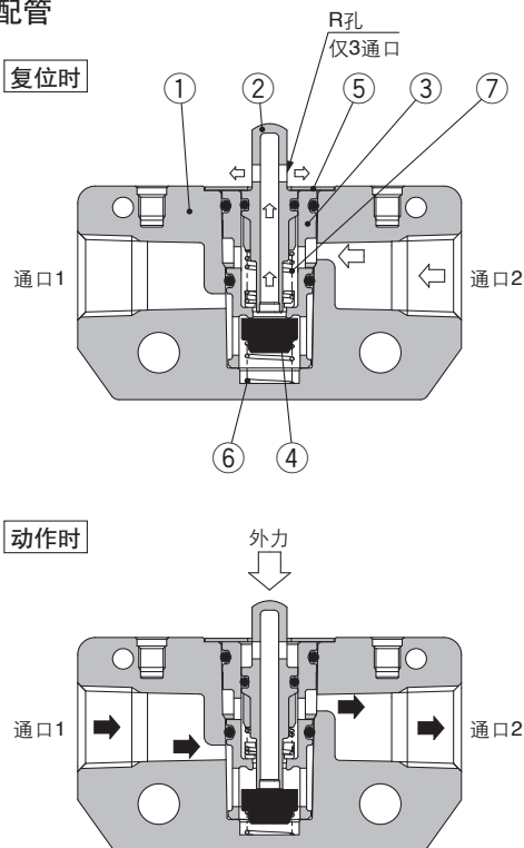
侧向配管
